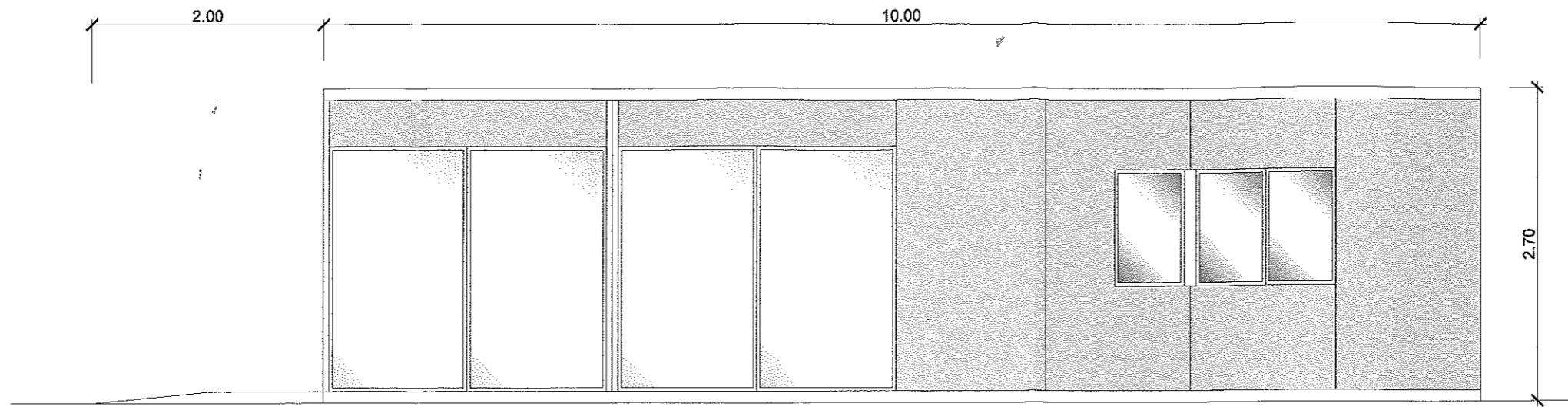
ALZADO 1 Escala 1:50
