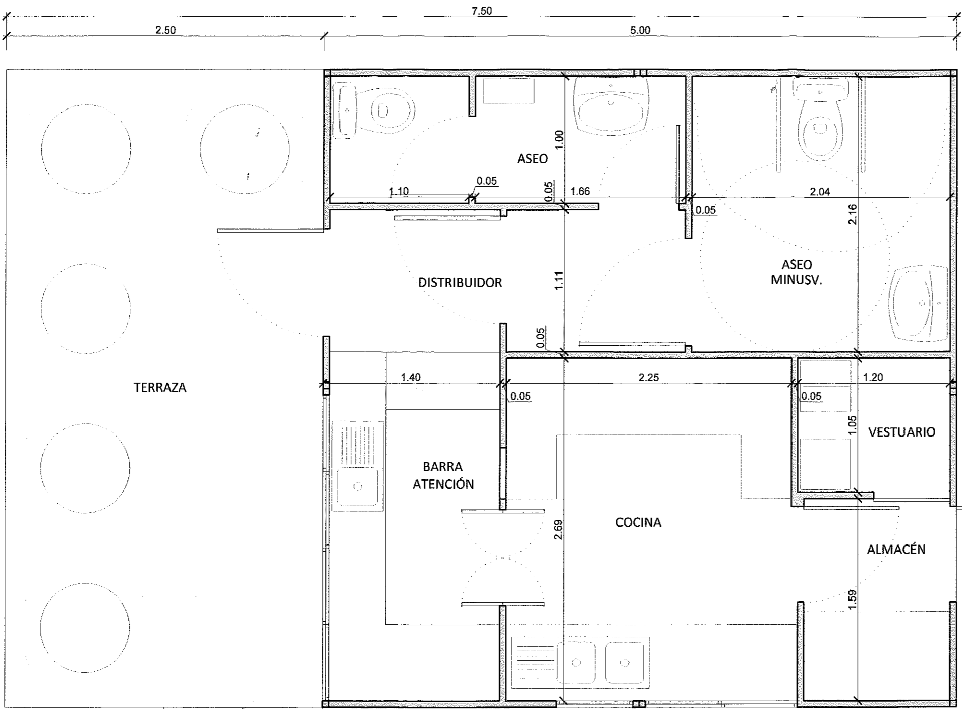
PLANTA SUELO: DISTRIBUCIÓN Y COTAS escala 1:30
