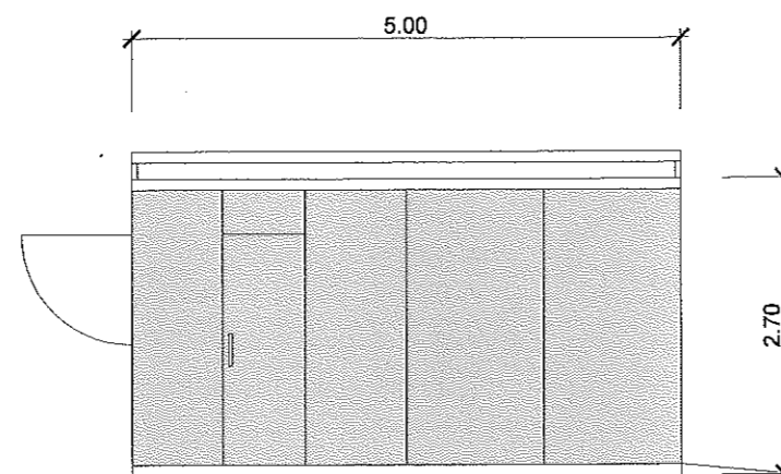
ALZADO 4 Escala 1:75
