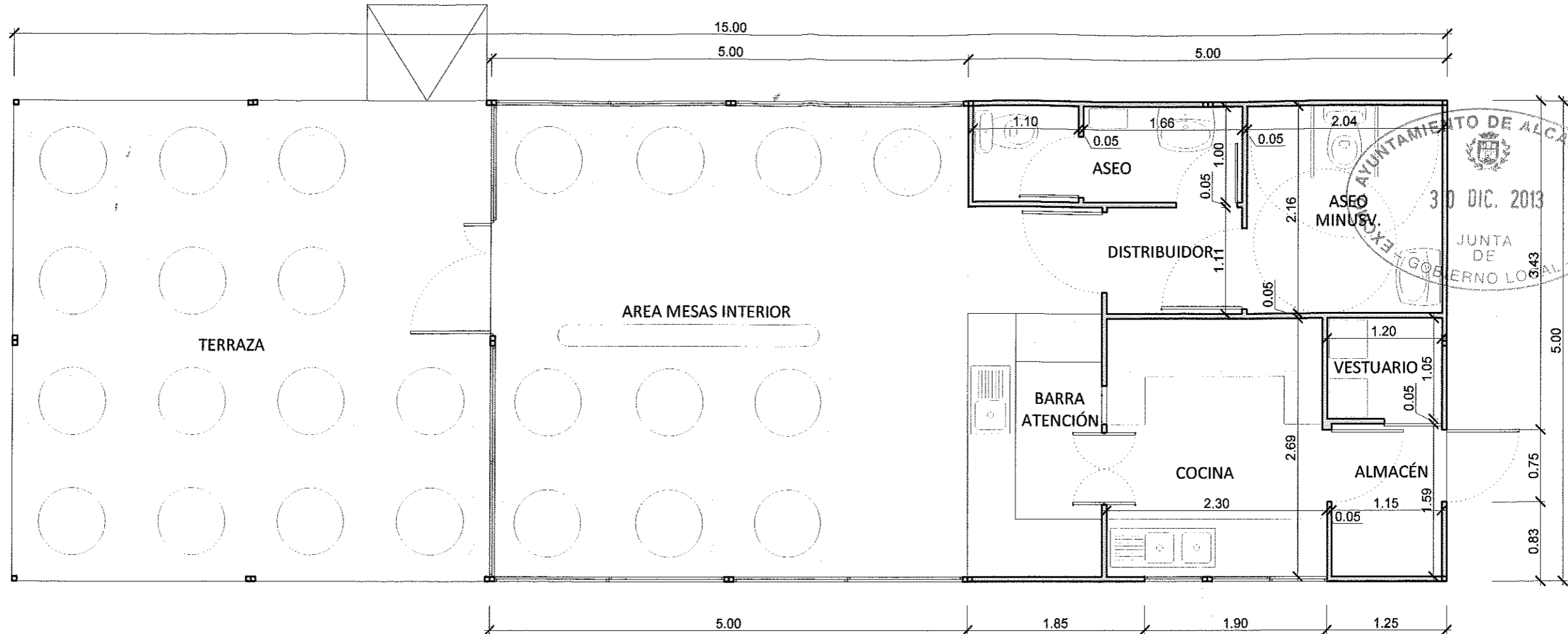
PLANTA SUELO: DISTRIBUCIÓN Y COTAS escala 1:50
