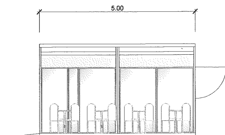
ALZADO 2 Escala 1:50
