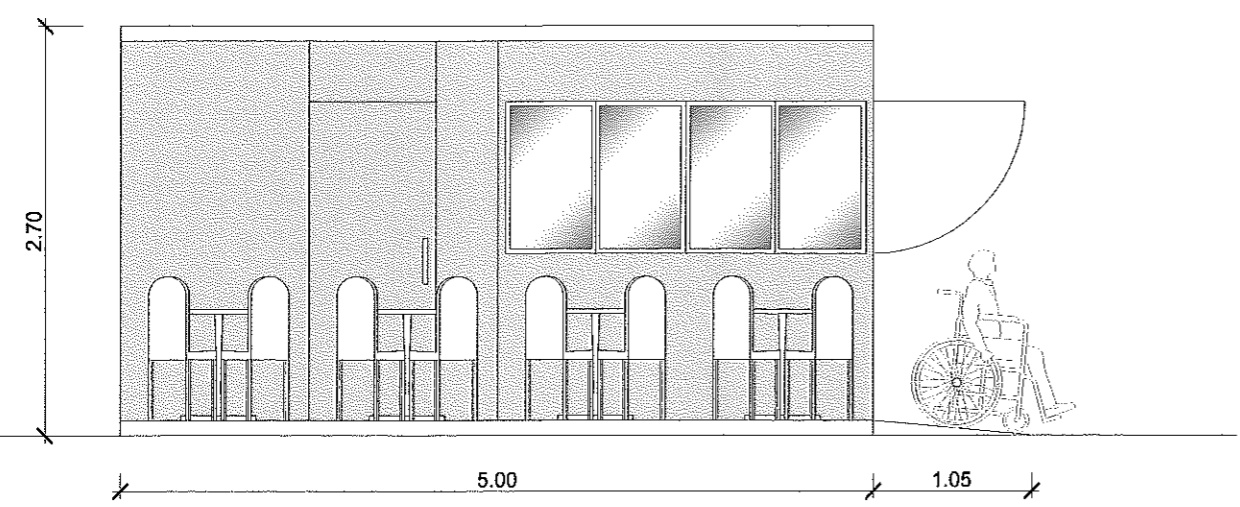
ALZADO 3 Escala 1:50
