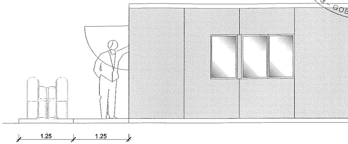
ALZADO 2 Escala 1:50
