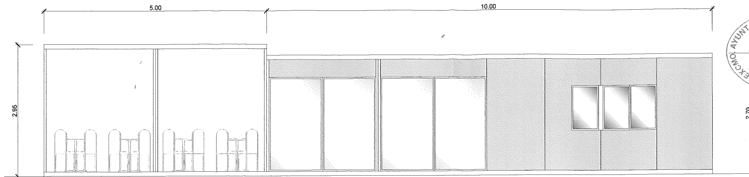
ALZADO 1 Escala 1:50
