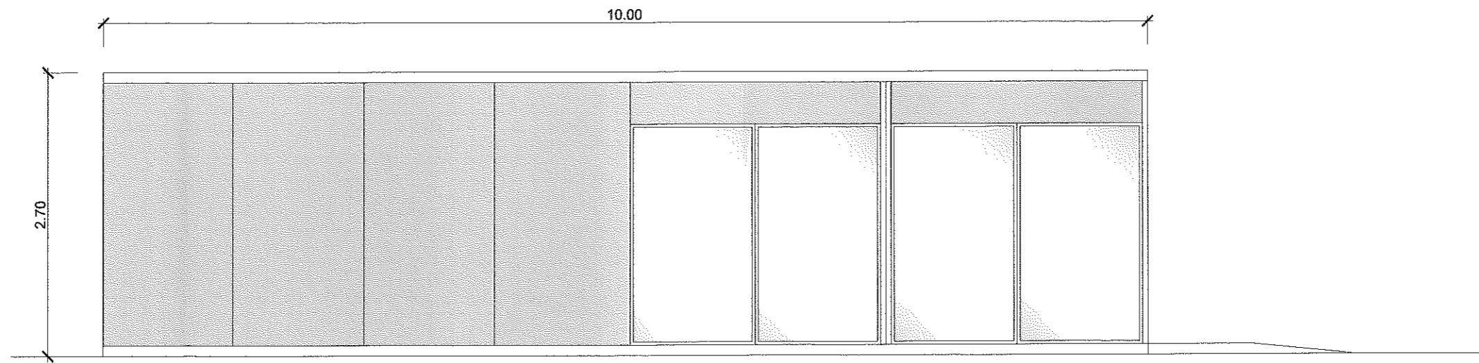
ALZADO 2 Escala 1:50
