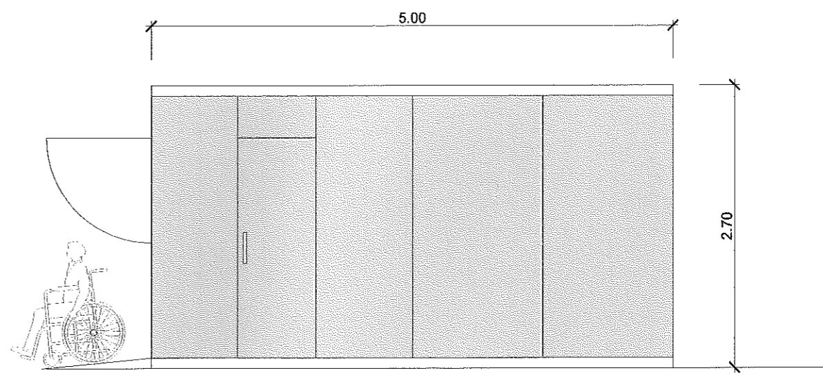
ALZADO 4 Escala 1:50
