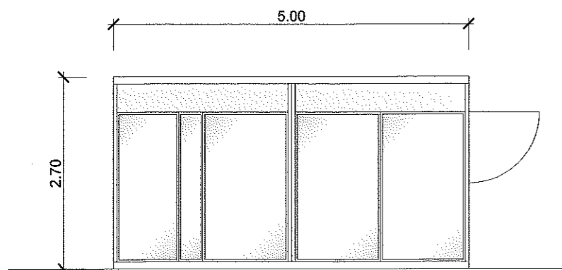
ALZADO 3 Escala 1:75
