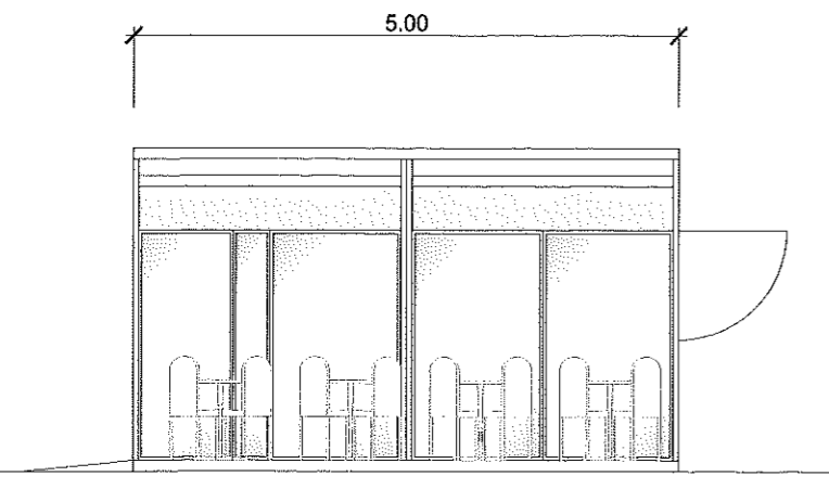
ALZADO 2 Escala 1:50
