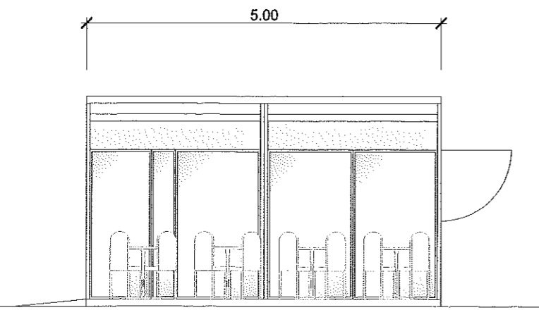
ALZADO 2 Escala 1:50
