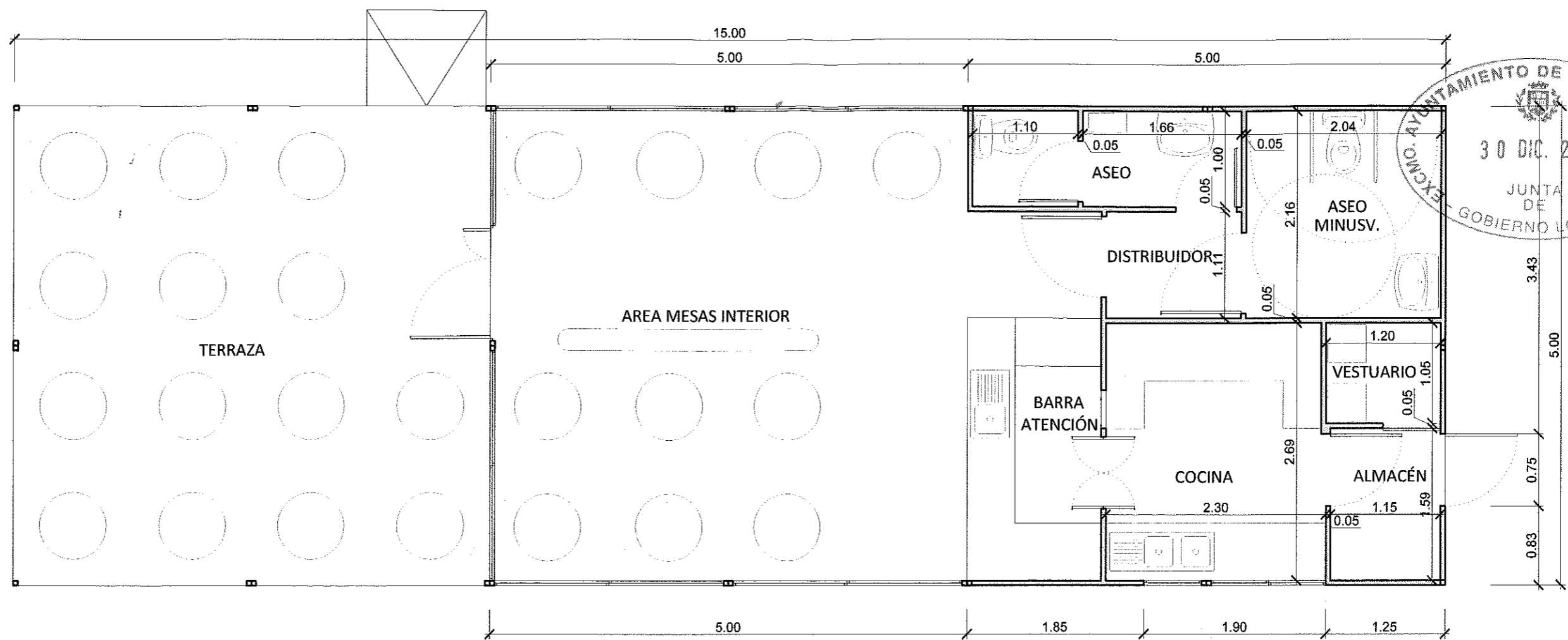
PLANTA SUELO: DISTRIBUCIÓN Y COTAS escala 1:50
