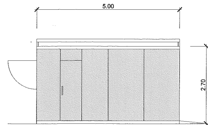
ALZADO 4 Escala 1:75
