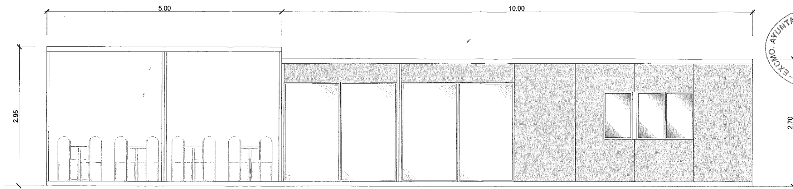
ALZADO 1 Escala 1:50
