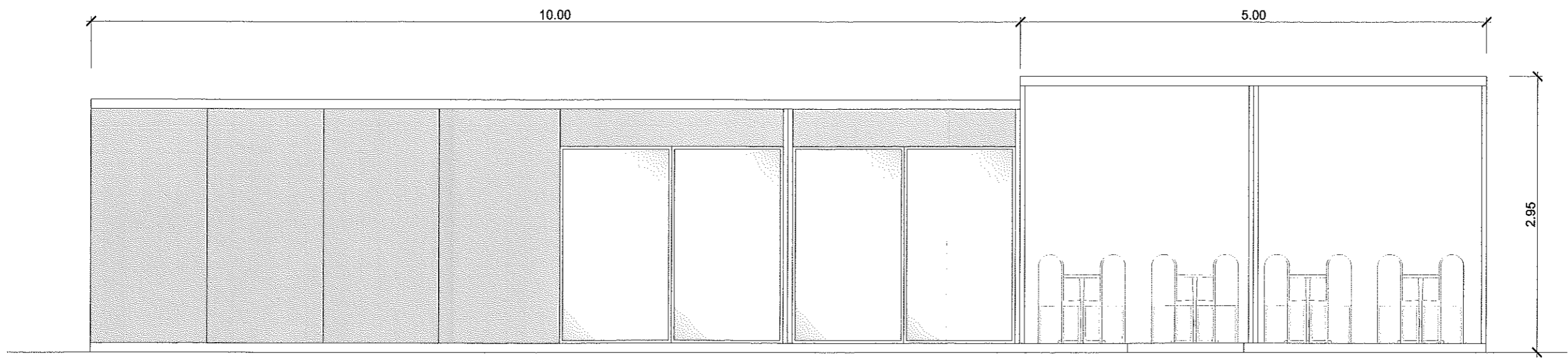
ALZADO 2 Escala 1:50
