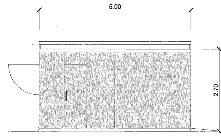
ALZADO 4 Escala 1:75
